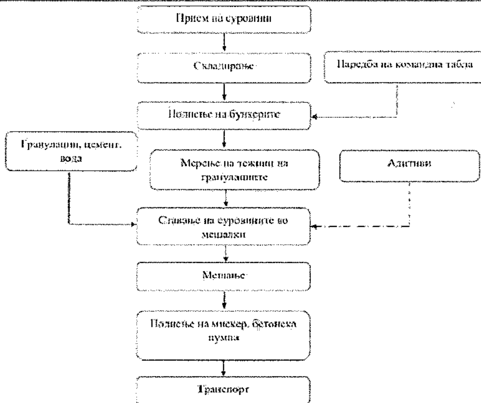
Слика 1. Дијаграм на технолошкиот процес на производство на бетон
