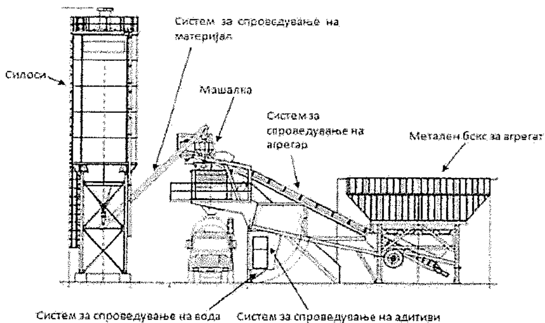
Слика 3. Шематски приказ на опремата во бетонската база технолошкиот процес на производство на бетон
