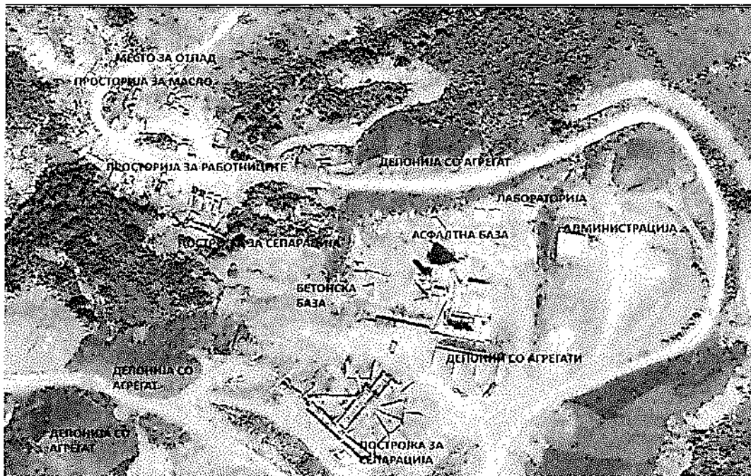
Слика 4. Распоред на објекти и опрема на МИСА-МГ ТРАНСПОРТ ДОО Скопје и МИСА-МГ ДОО СКОПЈЕ на локацијата и пошироката околина
