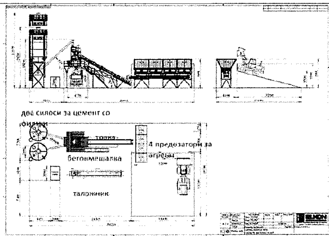
Слика 2а. Шематски приказ на технолошкиот процес на производство на бетон
